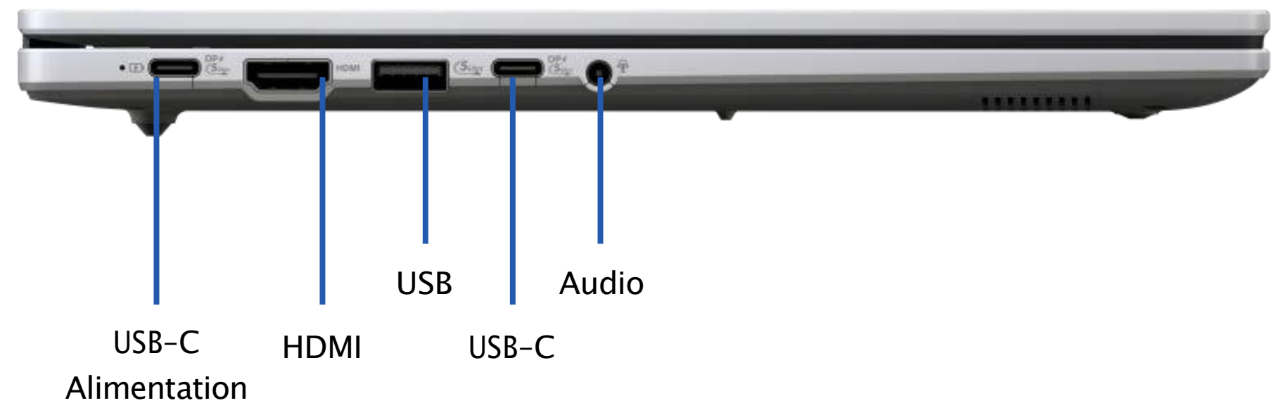
Vue gauche
